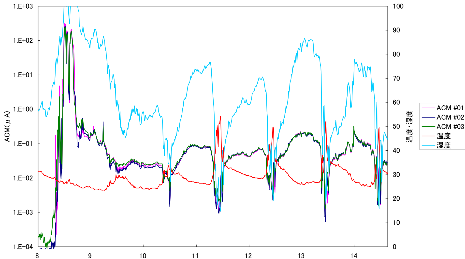
実暴露での弊社ACMセンサ出力比較
